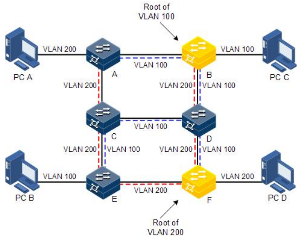
图 9-15 MST 域内多生成树实例组网示意图
