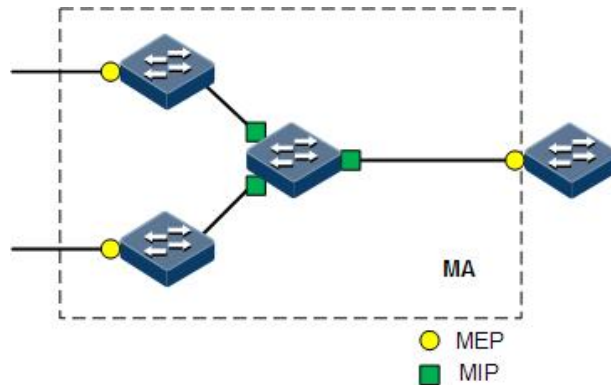
图 7-7 不同级别 MD 网络示意图
