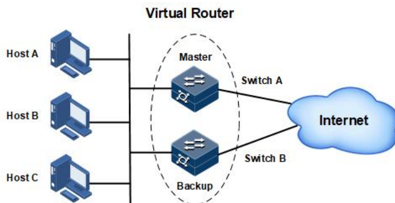
图 7-3 VRRP 原理示意图
