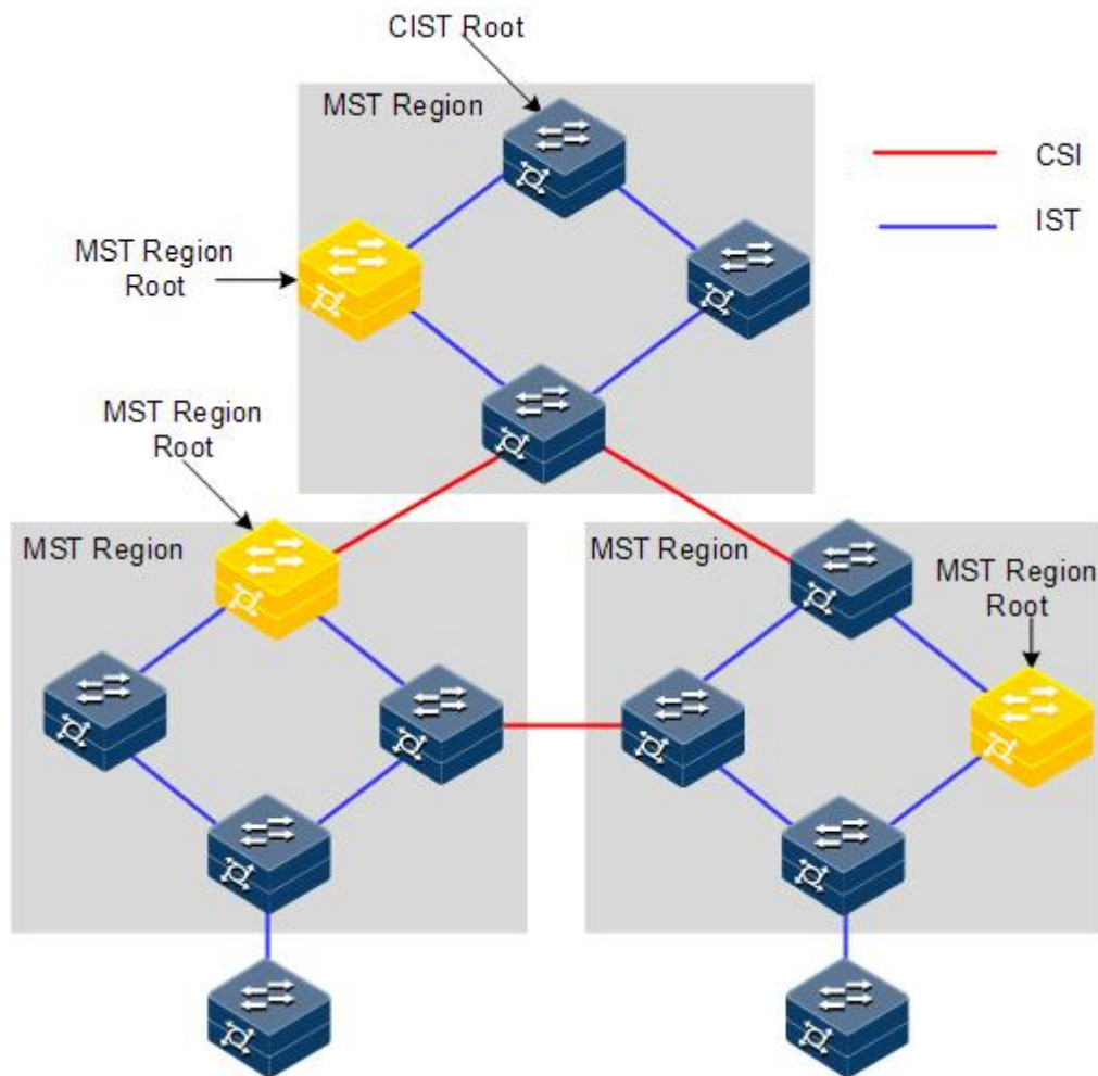
图 9-13 MSTP 网络基本概念示意图
