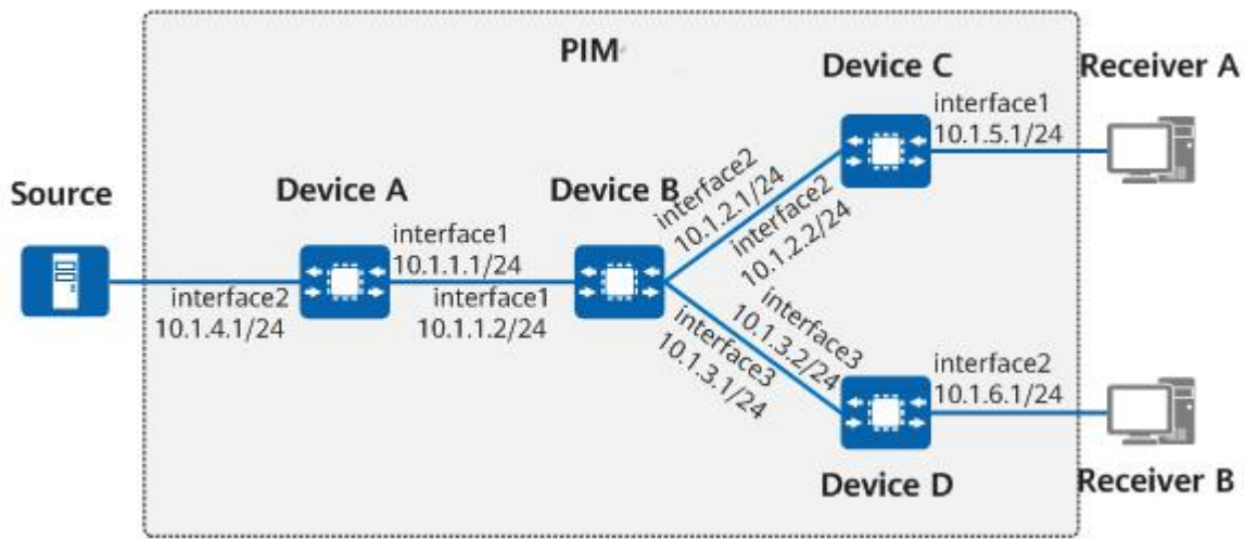
图 6-20 PIM-DM 功能功能组网应用示意图
