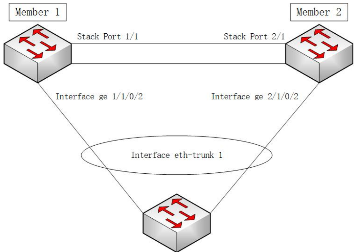
图 10-20 MAD 代理模式
