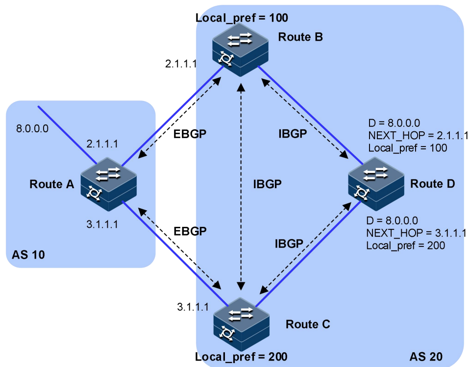
图 3-9 LOCAL_PREF 属性
