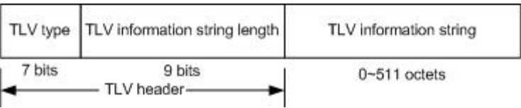
图 10-8 基本 TLV 结构图
