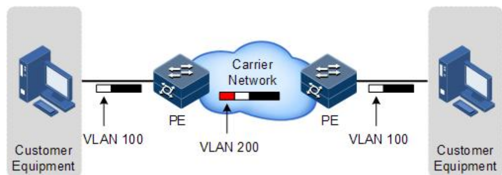
图 2-6 基本 QinQ 典型组网示意图
