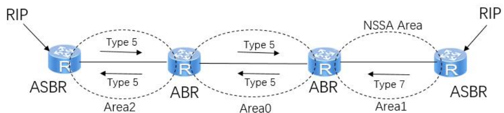
图 3-38 OSPFV3 NSSA 区域示意图
