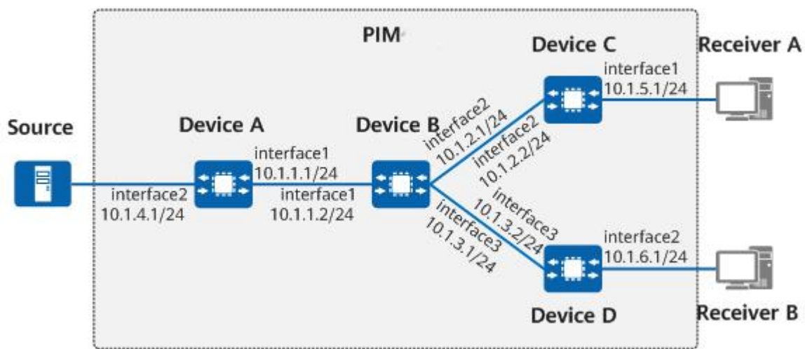
图 6-21 PIM-SM 功能功能组网应用示意图
