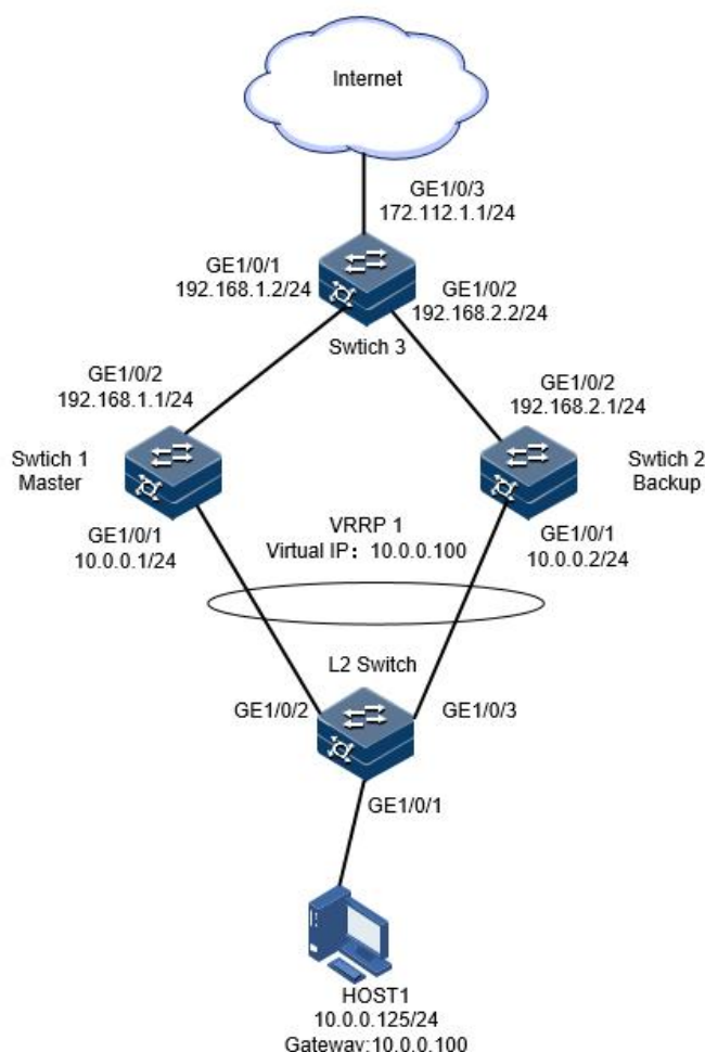
图 7-5 配置 VRRP 主备组网图
