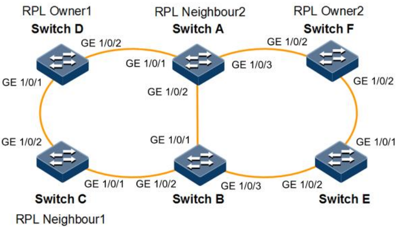
图 9-8 相交环 G.8032 应用组网示意图
