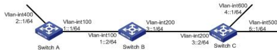
图 3-47 RIPng 基本功能组网图
