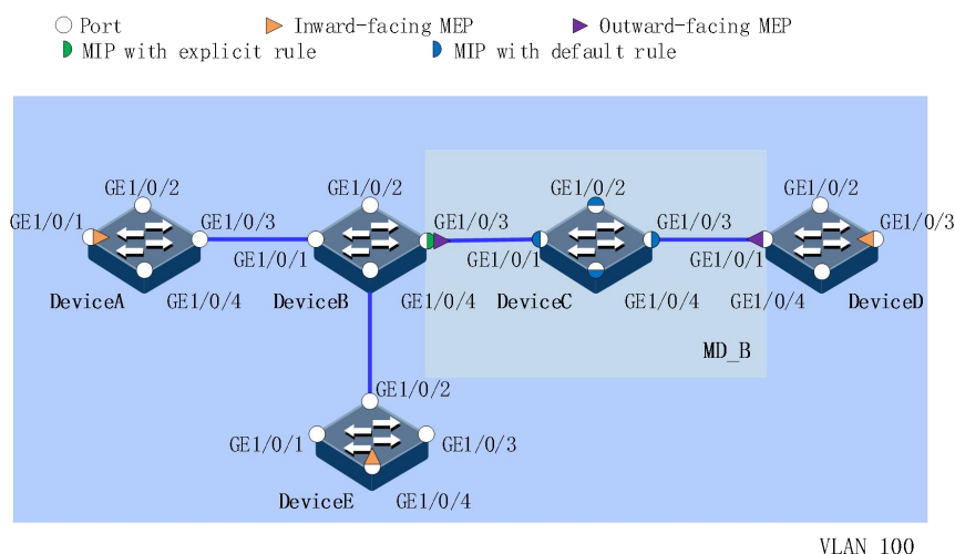
图 7-8 CFM 典型配置组网图
