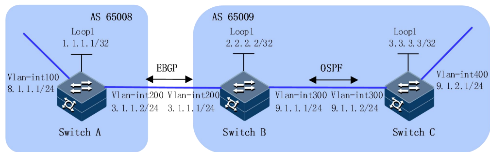
图 3-14 BGP 与 IGP 交互配置组网图
