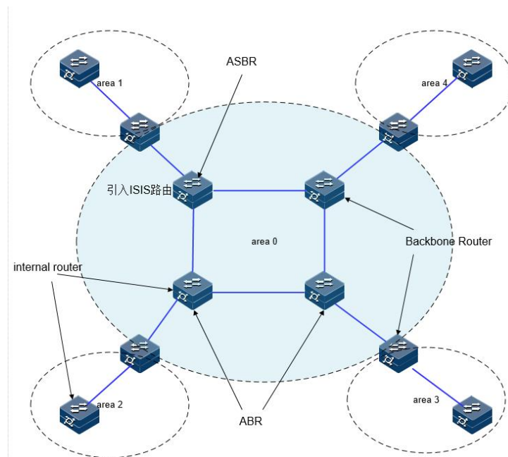
图 3-21 OSPF 路由器类型示例
