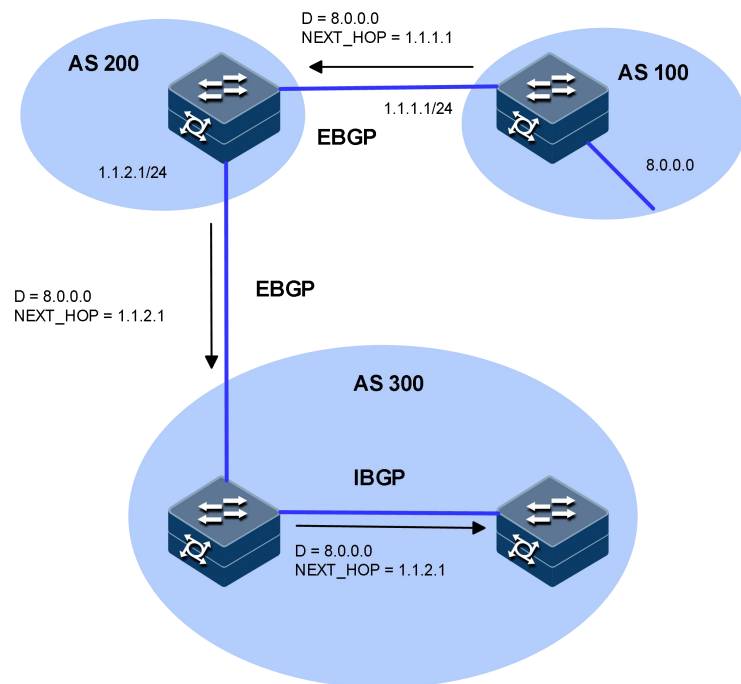
图 3-7 NEXT_HOP 属性
