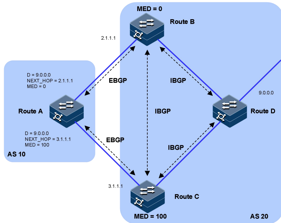
图 3-8 MED 属性
