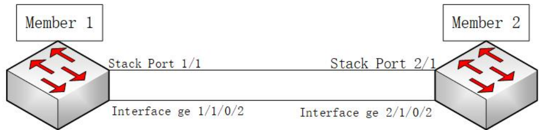
图 10-19 MAD 直连模式
