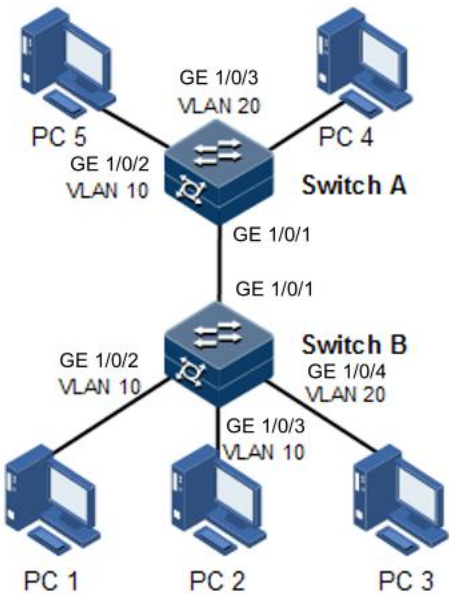
图 2-4 VLAN 和接口保护组网示意图
