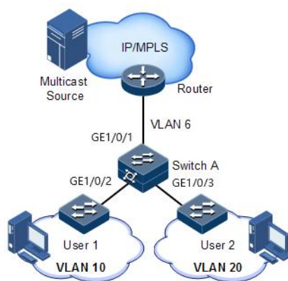
图 6-14 MLD Snooping 组播复制功能组网应用示意图
