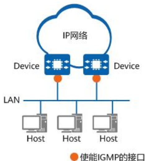
图 6-17 IGMP 在组播网络中的部署位置
