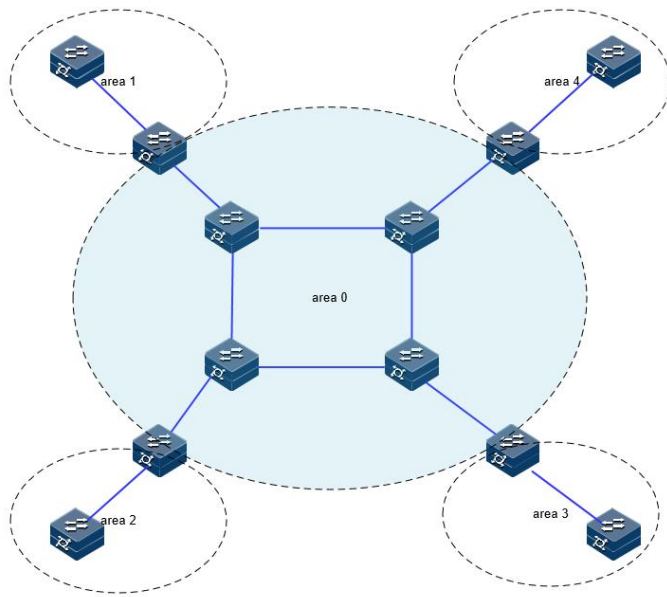
图 3-20 OSPF 区域划分
