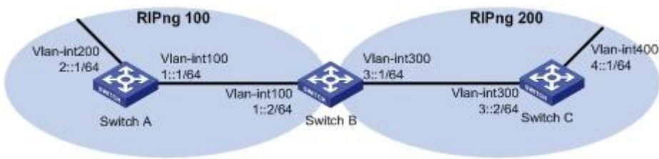
图 3-48 RIPng 引入外部路由组网图
