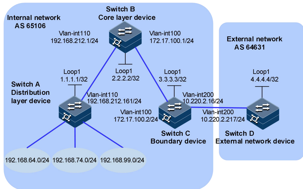
图 5-15 BGP 路由聚合组网图
