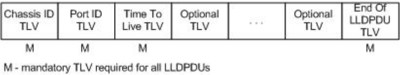
图 12-7 LLDPDU 结构图
