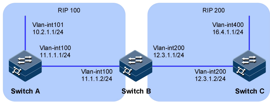
图 5-46 RIP 引入外部路由配置组网图
