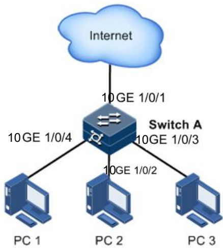
图 11-18 接口保护组网示意图
