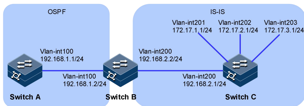
图 5-49 ipv4 路由引入中应用路由策略组网图
