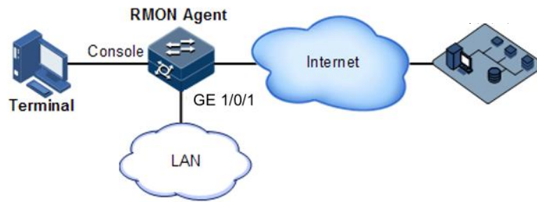
图 12-6 RMON 典型应用组网示意图
