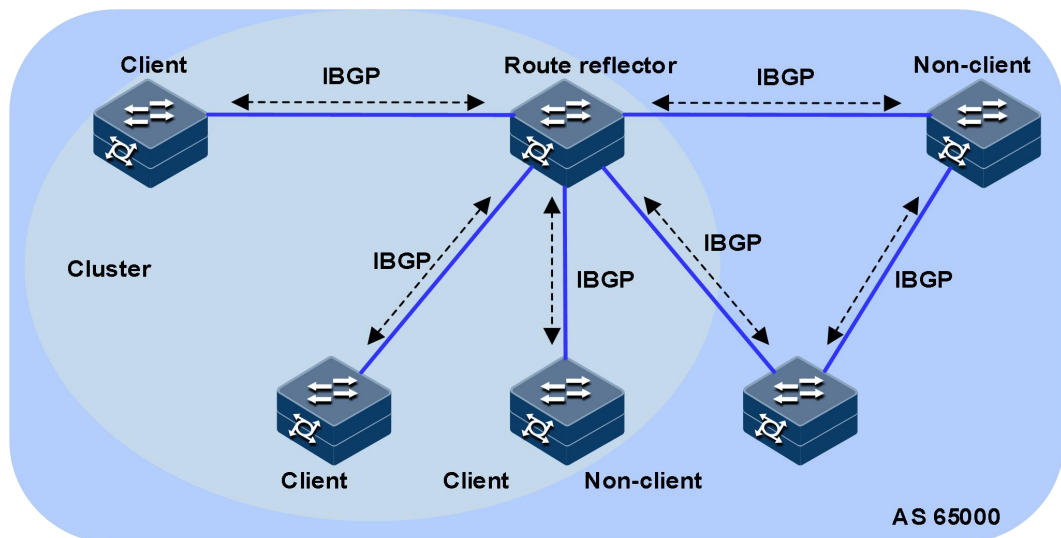
图 5-11 BGP 路由反射器示意图
