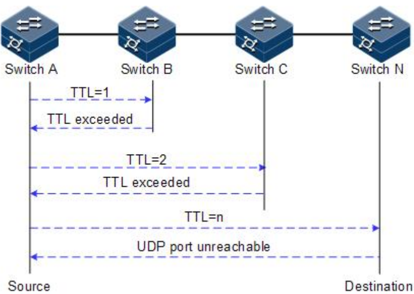
图 12-15 Trace 功能实现原理组网示意图
