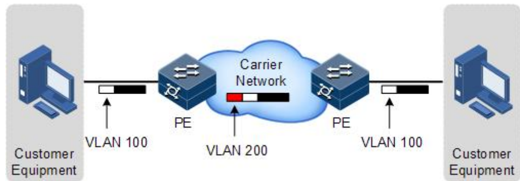
图 4-5 基本 QinQ 典型组网示意图
