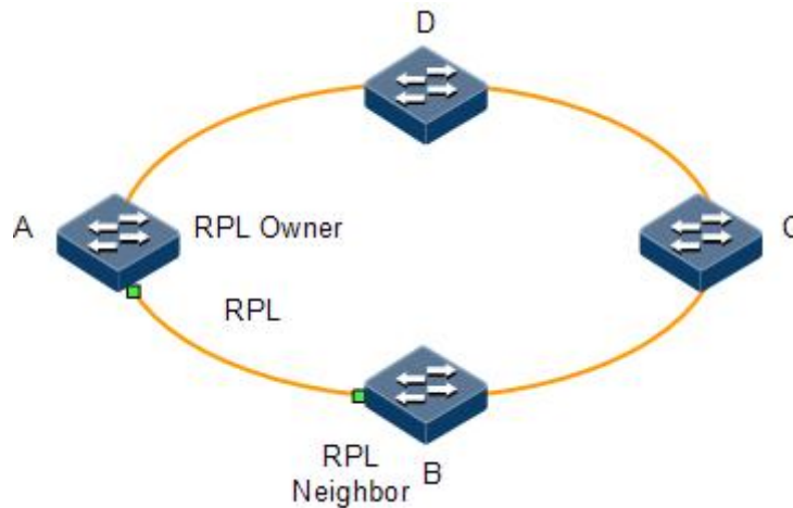
图 11-2 G.8032 环网示意图
