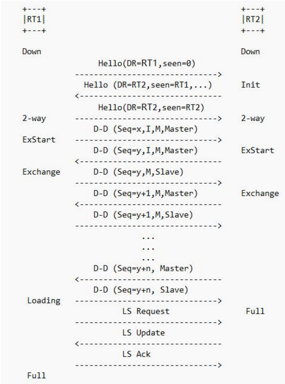
图 5-37 OSPFV3 广播网络建邻示意图
