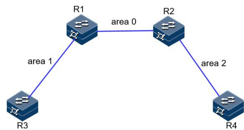
图 5-41 OSPFV3 NSSA 区域示例组网图
