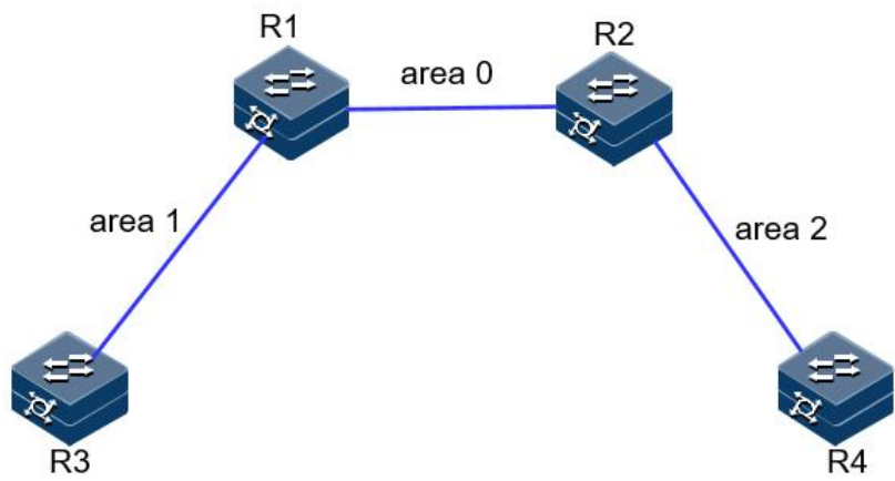
图 5-27 OSPF STUB 区域示例组网图
