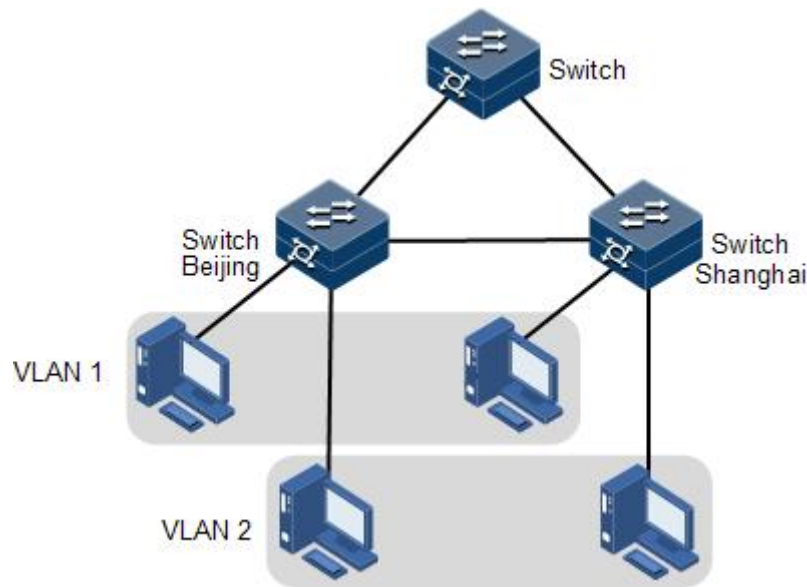
图 4-3 VLAN 划分示意图
