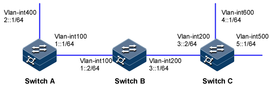
图 5-47 RIPng 基本功能组网图
