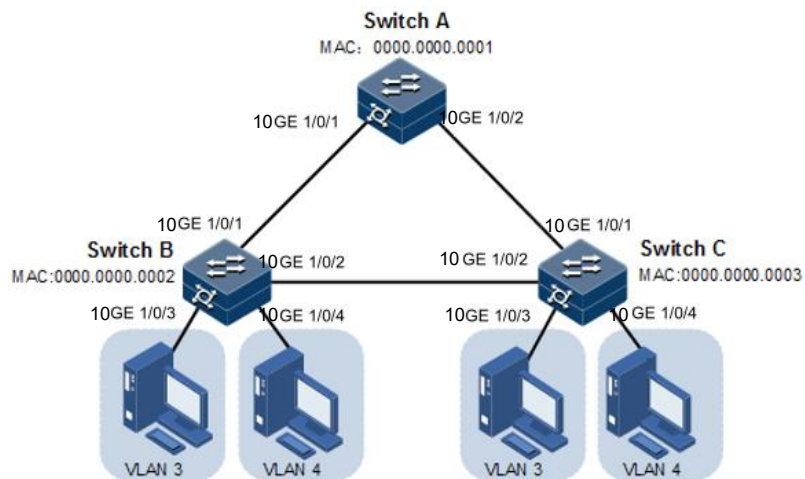
图 11-15 MSTP 应用组网示意图
