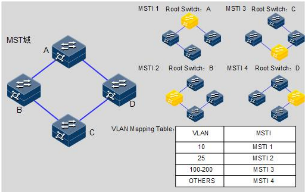
图 11-13 MSTI 概念示意图
