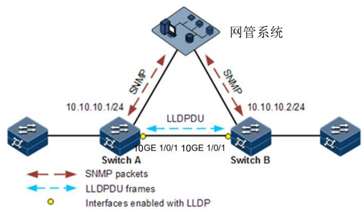
图 12-9 配置 LLDP 基本功能组网示意图
