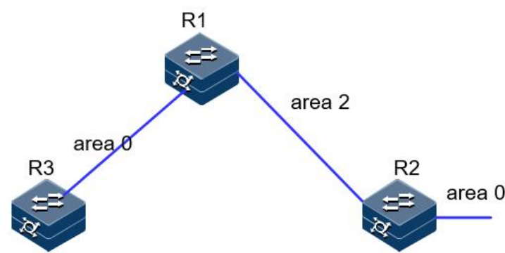
图 5-31 配置 OSPF 虚连接的组网图
