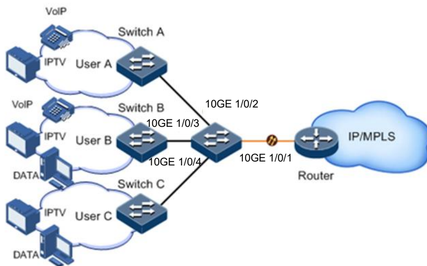
图 7-6 配置基于接口的流量限速组网示意图
