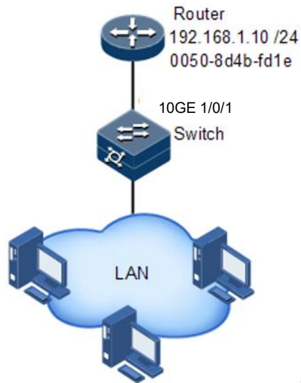
图 5-2 配置 ARP 组网示意图
