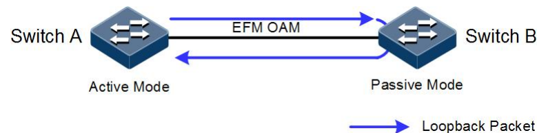
图 9-1 OAM 环回示意图
