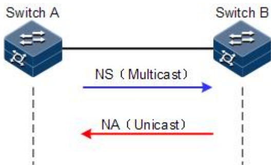
图 5-3 NDP 地址解析原理示意图
