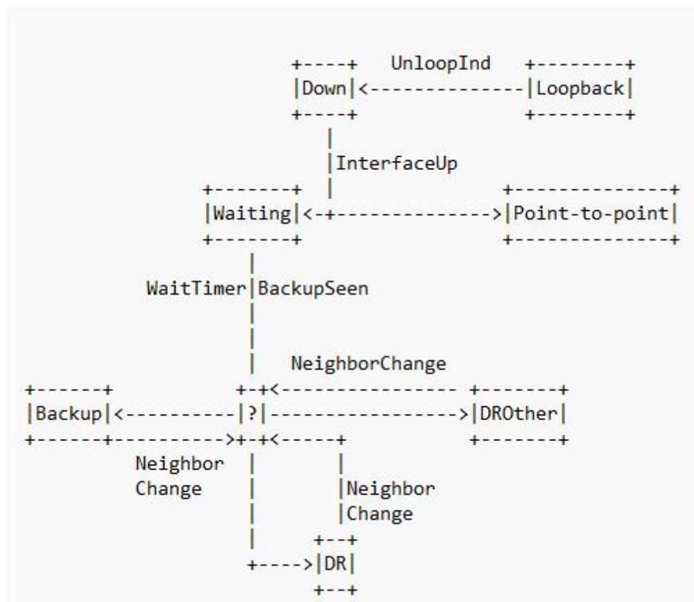
图 5-23 OSPF 接口状态机
