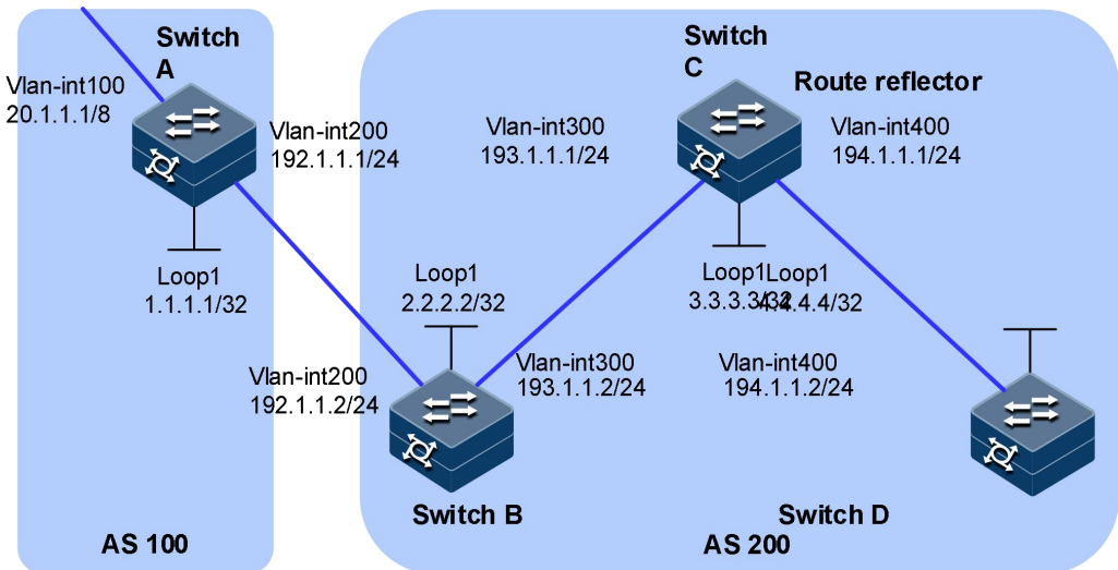
图 5-17 配置 BGP 路由反射器的组网图
