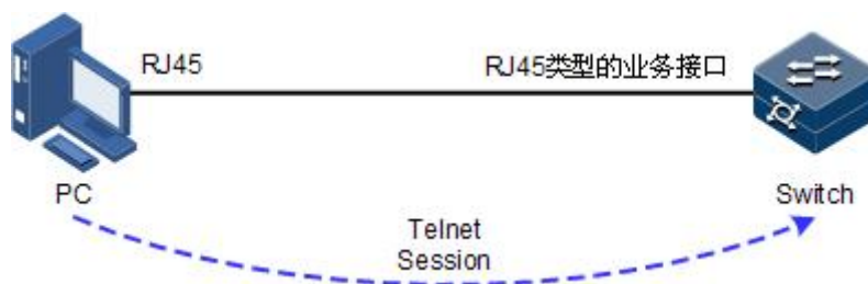
图 1-3 设备作为 Telnet Server 设备的组网示意图
