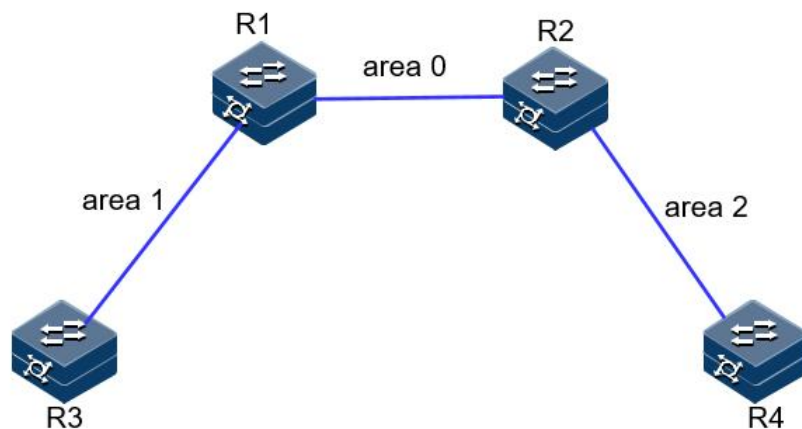
图 5-39 OSPFV3 基本配置组网图
