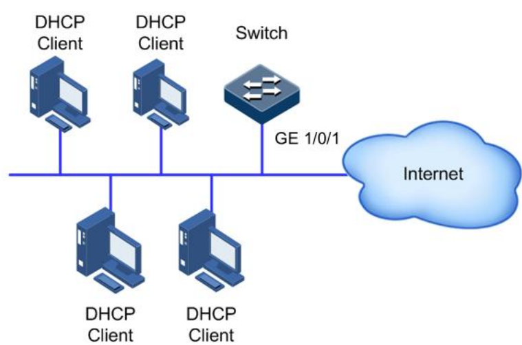
图 6-7 配置 DHCP 服务器组网示意图
