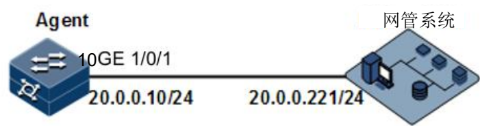
图 12-3 SNMP v1/v2c 组网示意图
