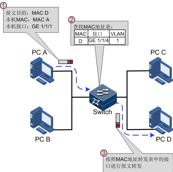
图 4-1 MAC 地址表转发示意图
