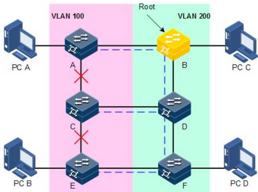
图 11-10 RSTP 协议造成 VLAN 报文无法转发示意图
