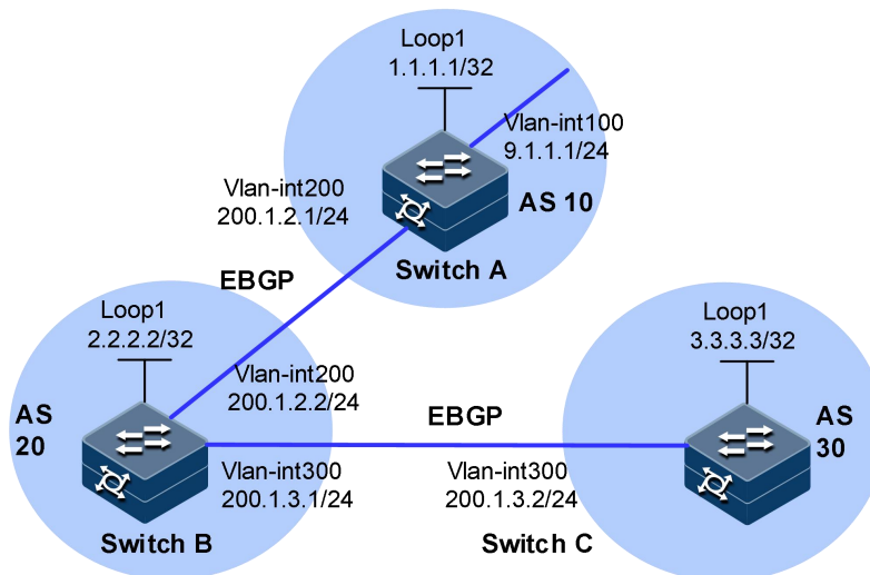
图 5-16 BGP 团体组网图
