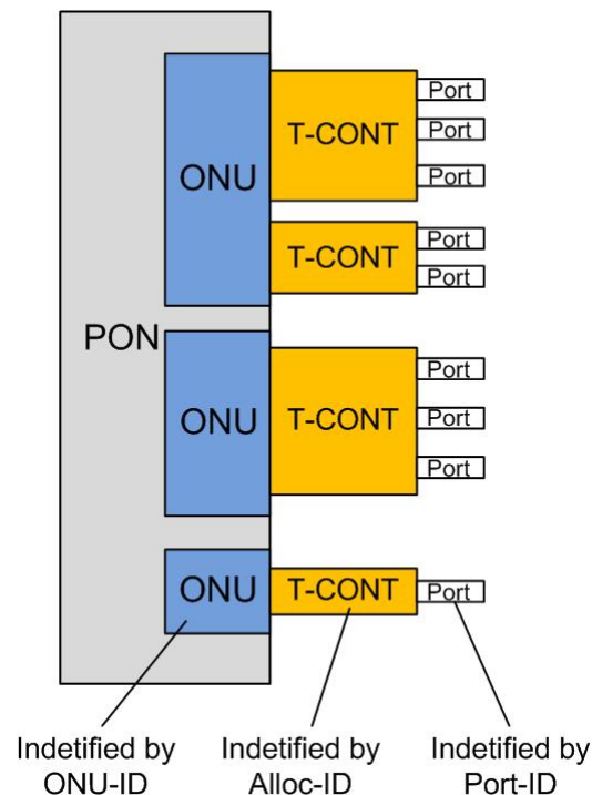
图 2-1 xPON 复用结构（GEM 方式）
