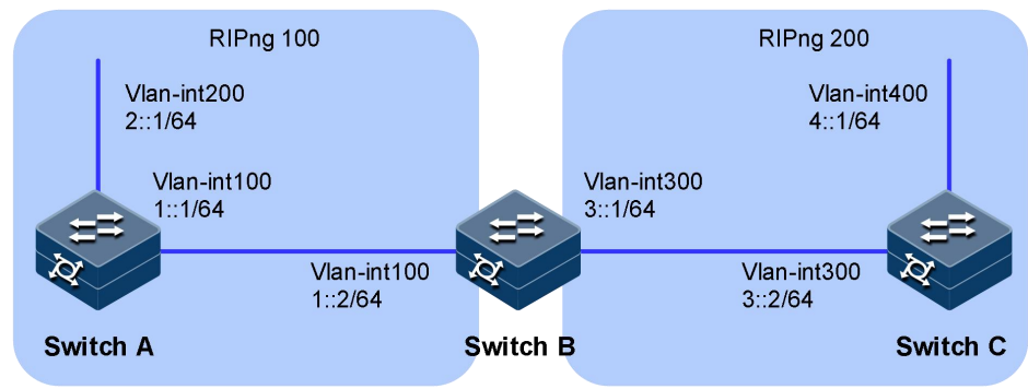
图 5-48 RIPng 引入外部路由组网图
