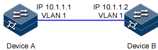
图 11-19 BFD 单跳应用
