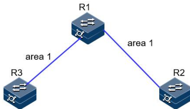
图 5-32 配置 OSPF 虚连接的组网图
