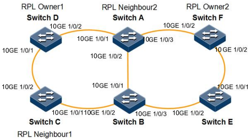
图 11-7 相交环 G.8032 应用组网示意图
