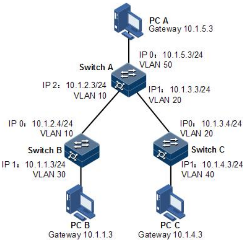
图 5-4 配置静态路由组网示意图
