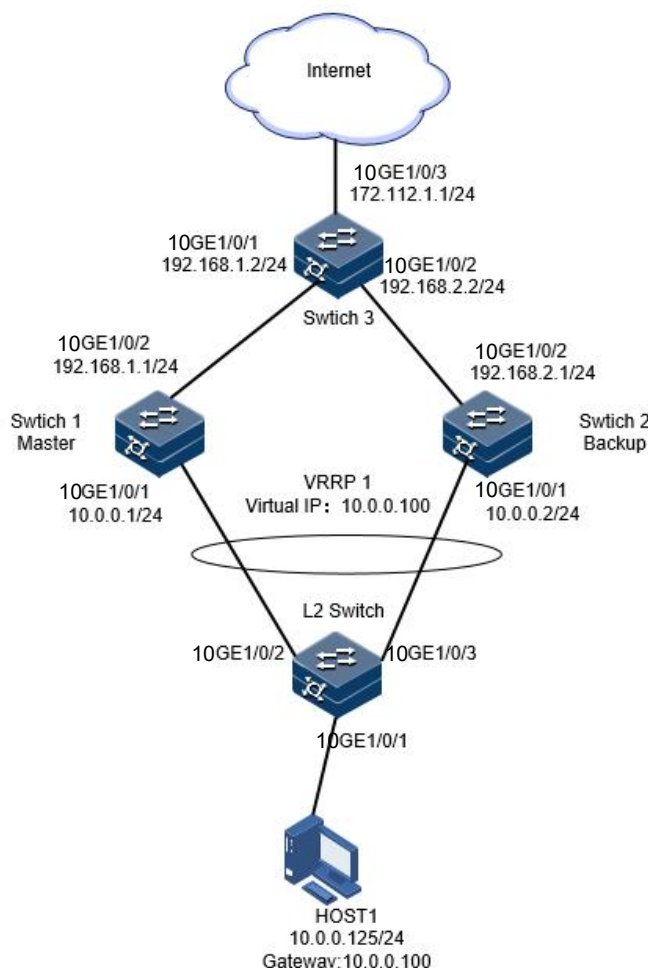
图 9-4 配置 VRRP 主备组网图
