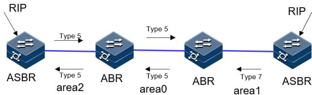
图 5-38 OSPFV3 NSSA 区域示意图
