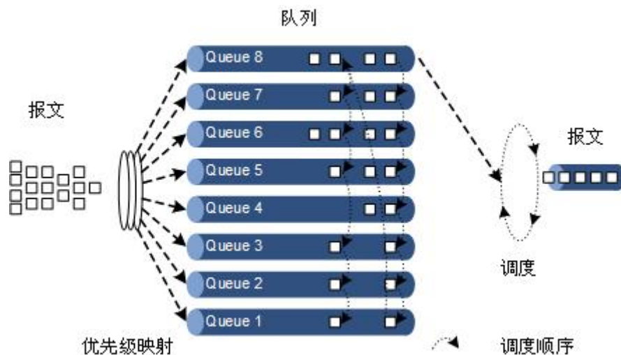
图 7-3 WRR 调度示意图
