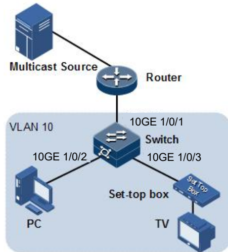
图 6-15 MLD Snooping Proxy 功能组网应用示意图
