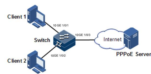
图 10-4 PPPoE+应用组网示意图
