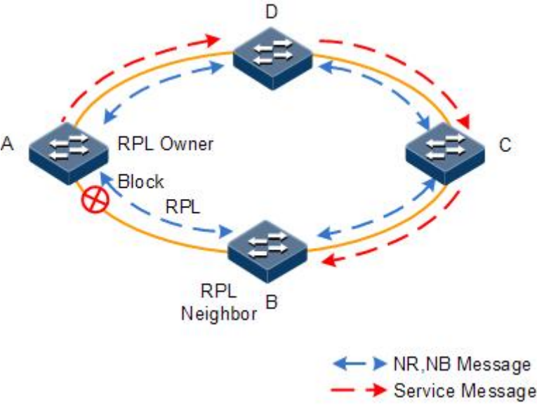
图 11-3 环网空闲状态
