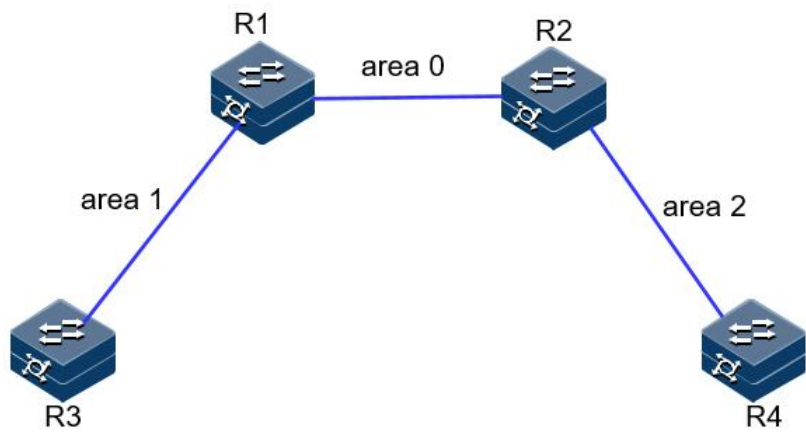
图 5-26 OSPF 基本配置组网图
