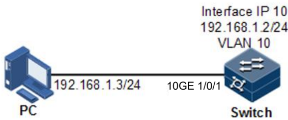
图 5-1 配置 VLAN 接口组网示意图
