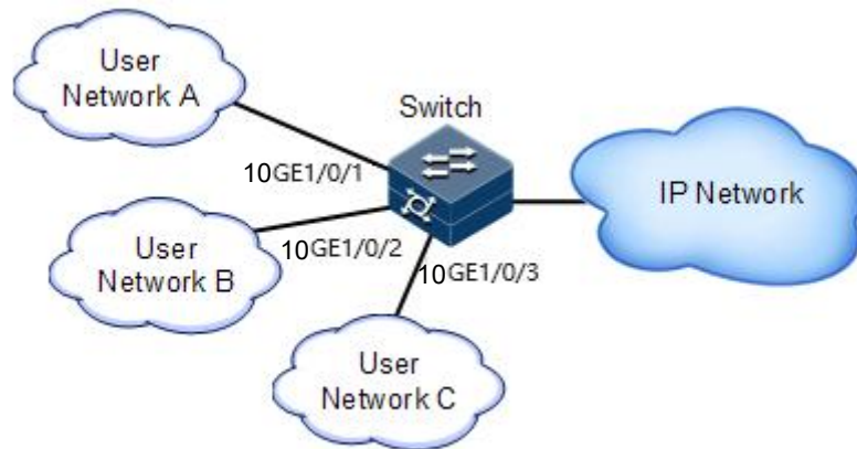
图 10-5 安全 MAC 应用组网示意图
