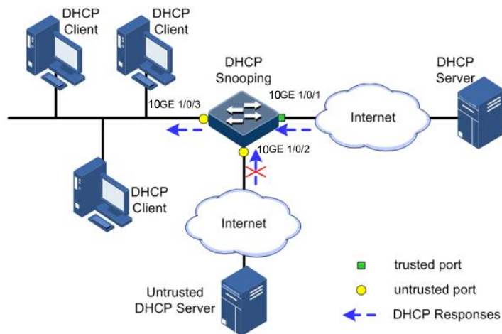
图 10-10 配置 DHCP Snooping 组网示意图
