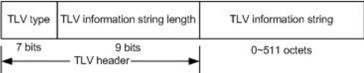
图 12-8 基本 TLV 结构图
