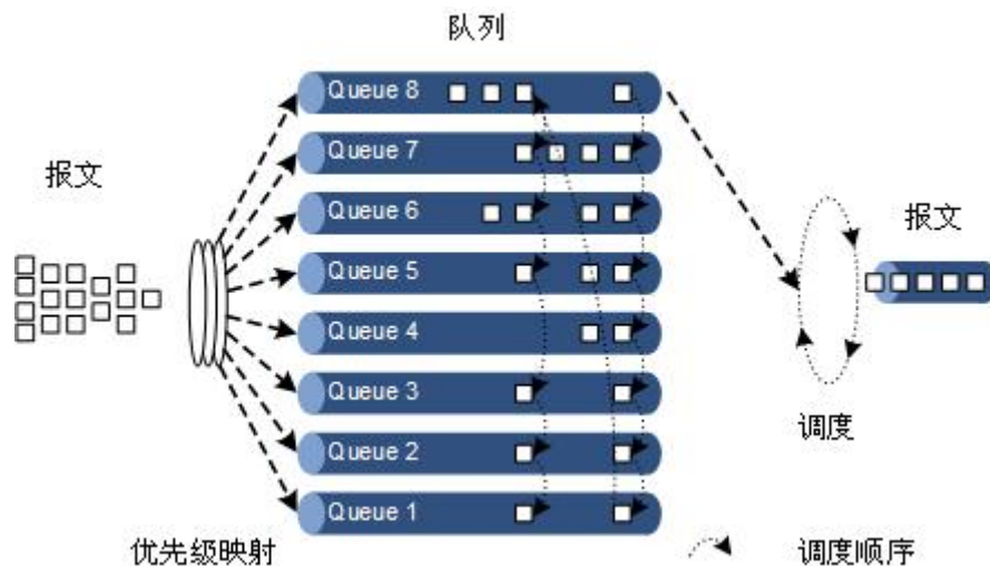
图 7-4 WFQ 调度示意图
