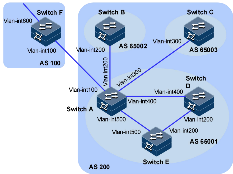
图 5-18 配置联盟组网图
