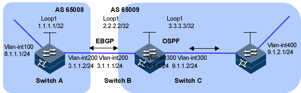
图 5-14 BGP 与 IGP 交互配置组网图
