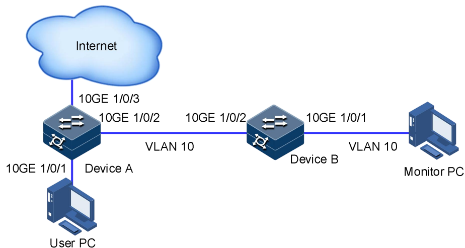
图 12-12 接口远端镜像应用组网示意图
