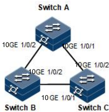
图 11-11 STP 应用组网示意图
