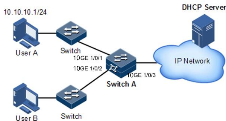
图 10-7 ARP 防攻击应用组网示意图
