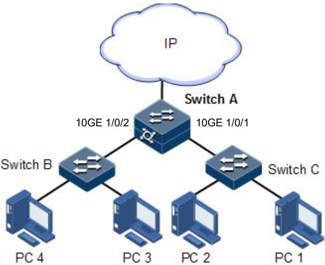
图 4-2 MAC 应用组网示意图
