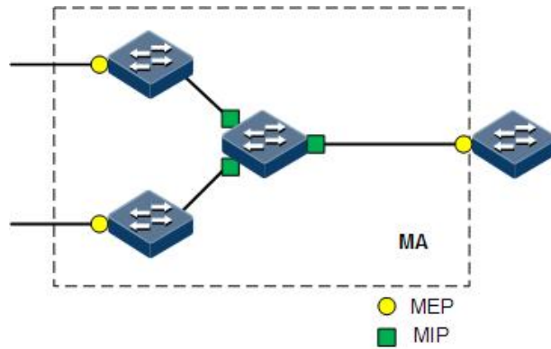
图 9-6 不同级别 MD 网络示意图
