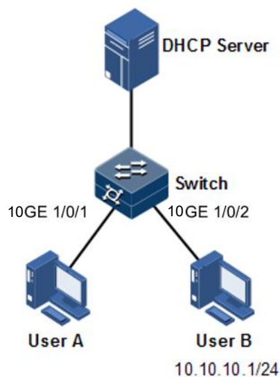
图 10-12 IP Source Guard 应用组网示意图
