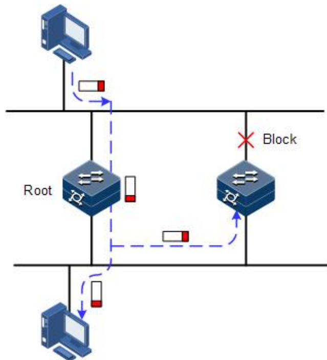
图 11-9 运行 STP 协议的环网示意图
