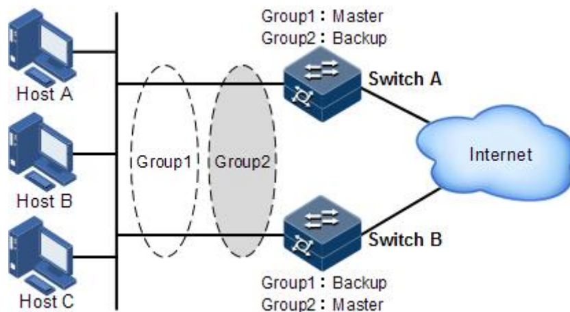
图 9-3 VRRP 负载分担原理示意图
