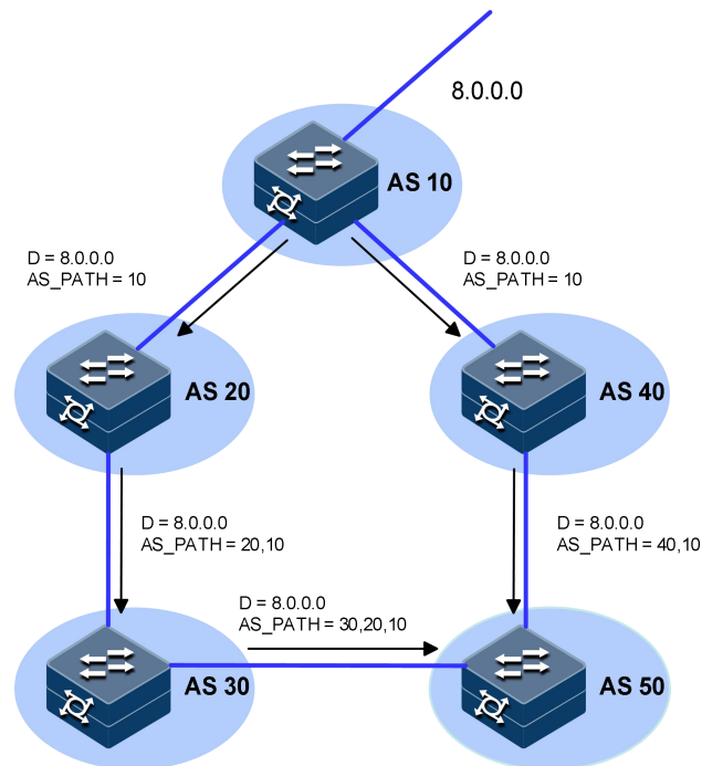
图 5-6 AS_PATH 属性
