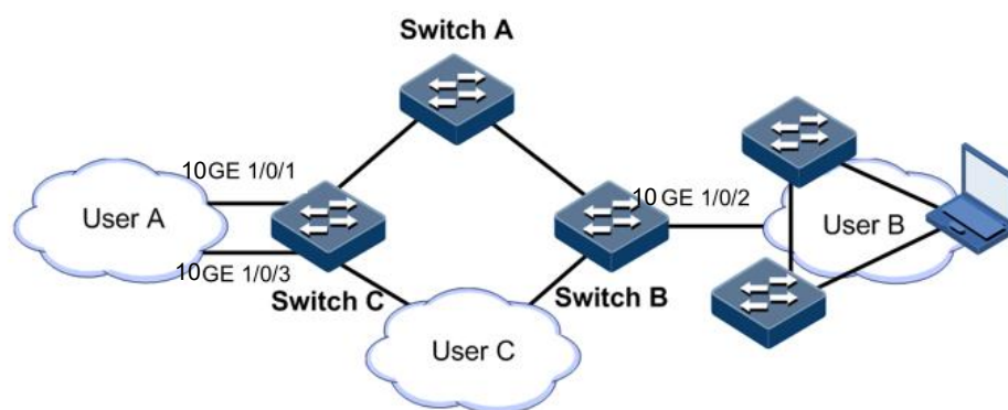
图 11-16 环路类型示意图
