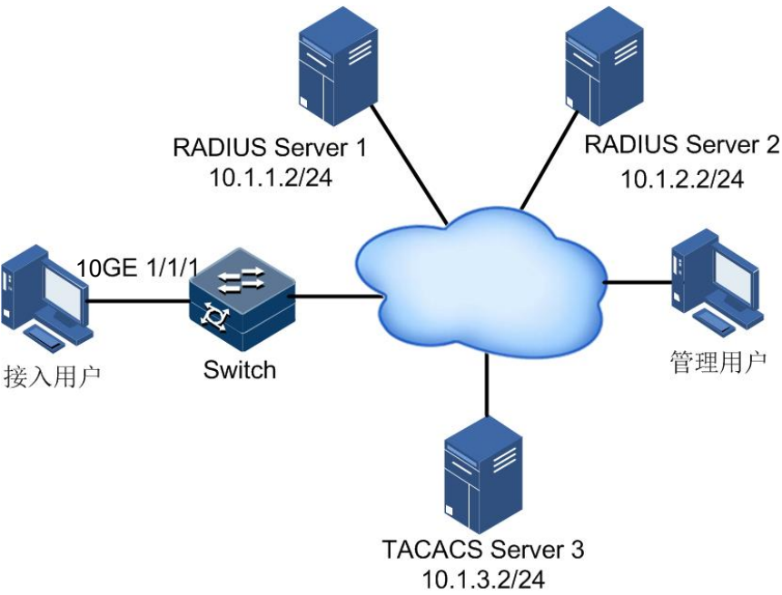
图 10-2 分域认证应用组网示意图
