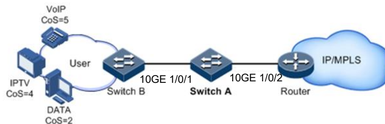
图 7-5 配置队列调度组网示意图
