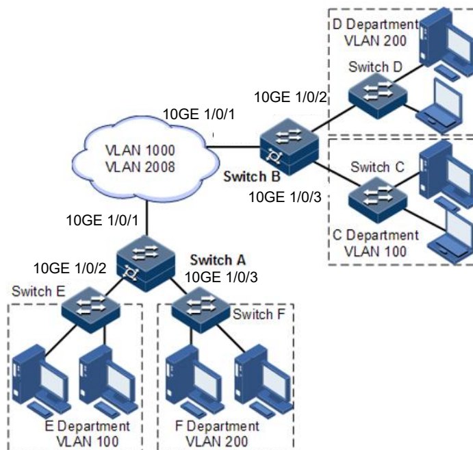
图 4-9 VLAN 转换应用组网示意图
