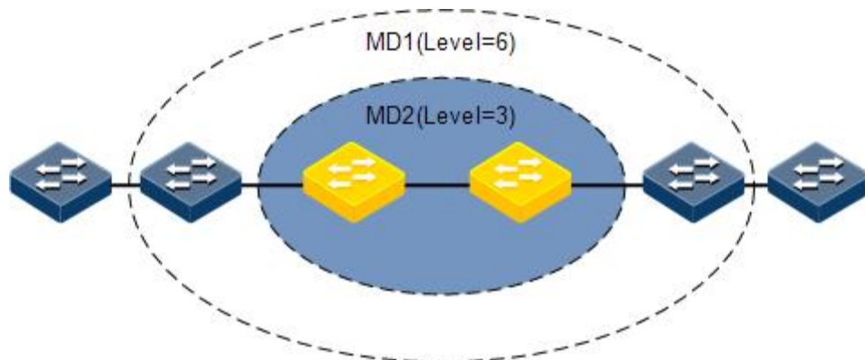
图 9-5 不同级别 MD 网络示意图
