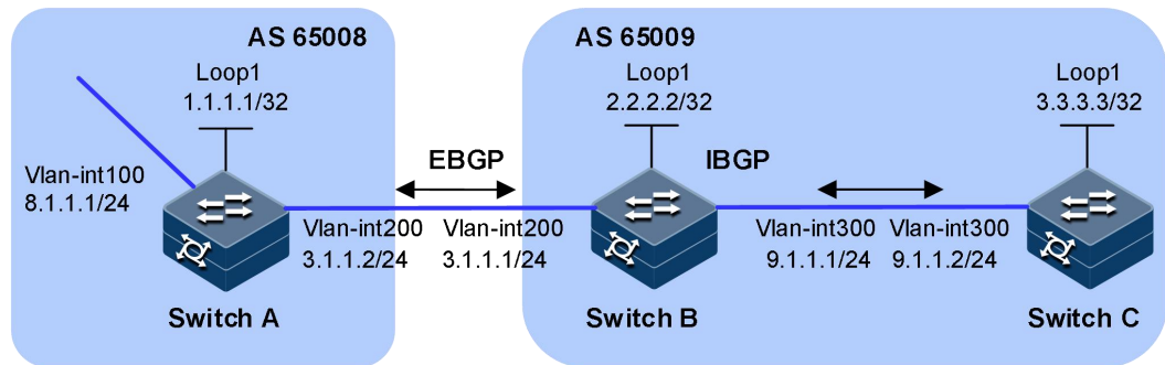
图 5-13 BGP 基本配置组网图
