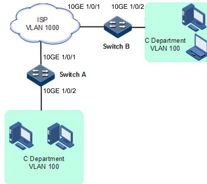
图 4-6 基本 QinQ 应用组网示意图
