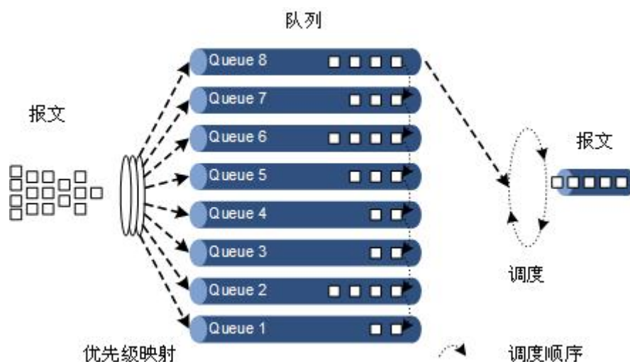
图 7-2 SP 调度示意图
