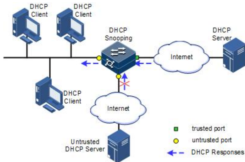
图 10-9 DHCP Snooping 组网示意图
