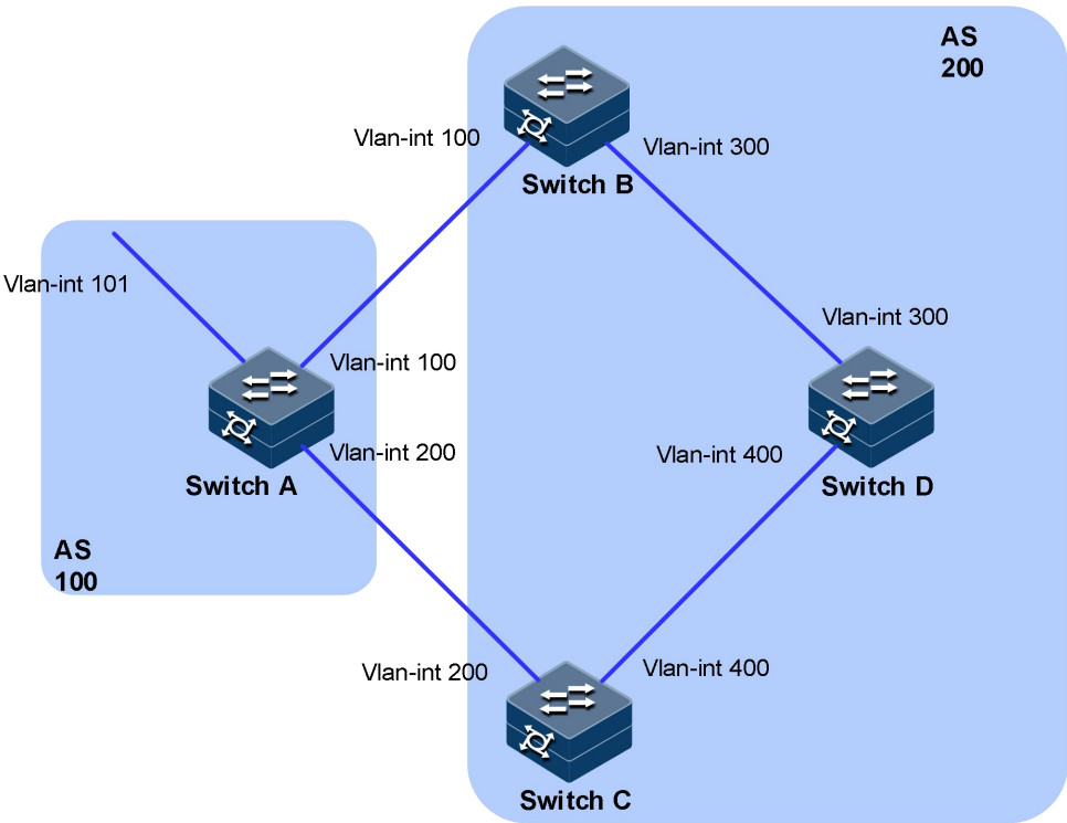
图 5-19 配置 BGP 路径选择的组网图
