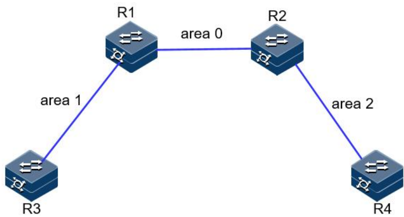
图 5-28 OSPF NSSA 区域示例组网图
