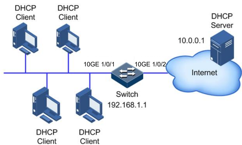
图 6-9 配置 DHCP 中继组网示意图
