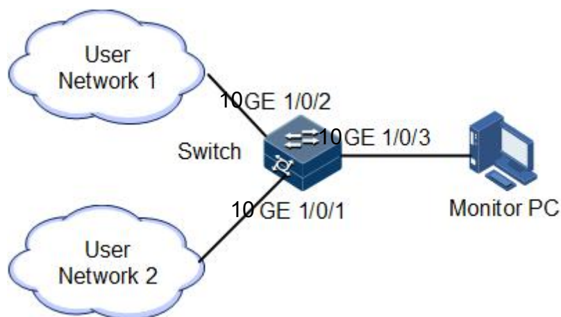
图 12-11 接口镜像应用组网示意图
