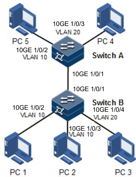
图 4-4 VLAN 和接口保护组网示意图
