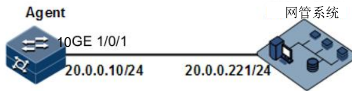
图 12-4 SNMP v3 和 Trap 组网示意图
