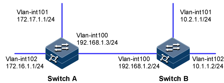
图 5-45 RIP 基本功能组网图
