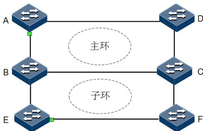
图 11-5 子环模型
