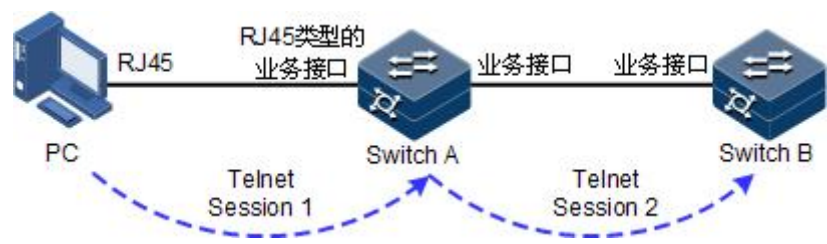
图 1-4 设备作为 Telnet Client 设备的组网示意图
