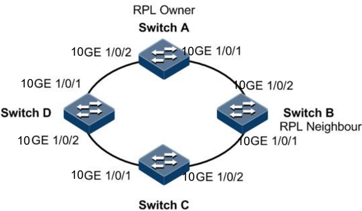
图 11-6 单环 G.8032 应用组网示意图
