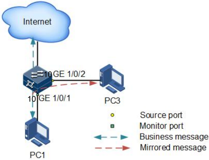
图 12-10 接口镜像功能原理示意图
