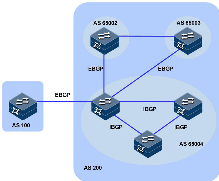
图 5-12 BGP 联盟示意图
