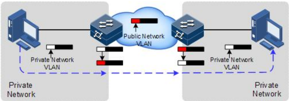
图 4-8 VLAN 转换原理组网示意图
