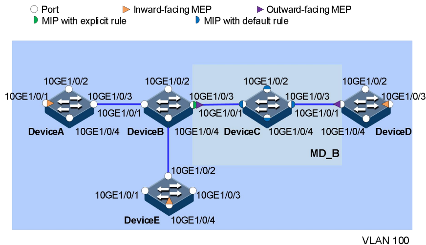
图 9-7 CFM 典型配置组网图
