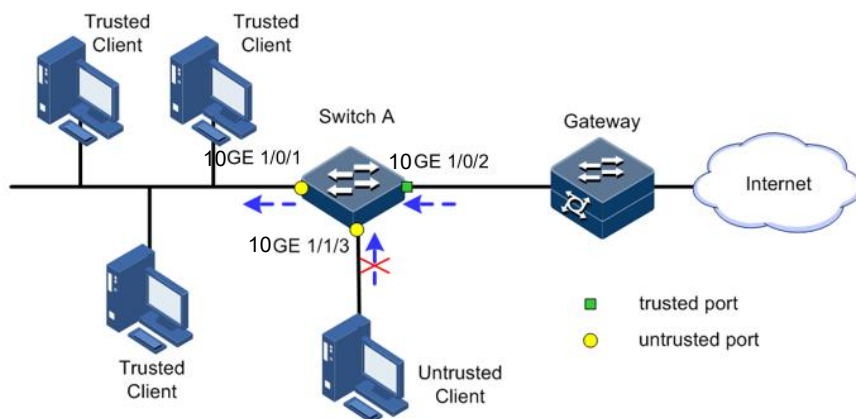
图 10-8 配置 ND Snooping 组网示意图
