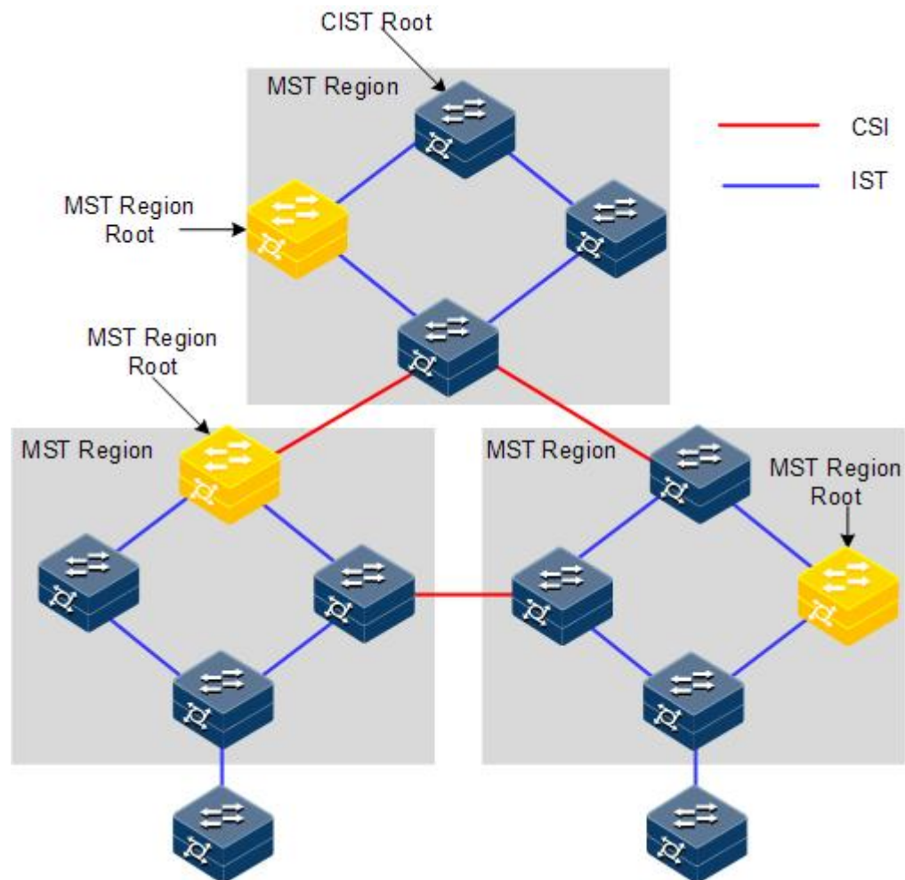
图 11-12 MSTP 网络基本概念示意图
