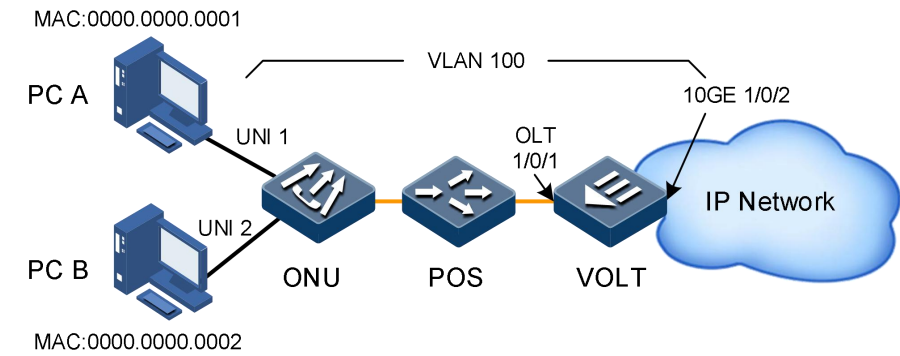
图 2-4 数据业务示例图
