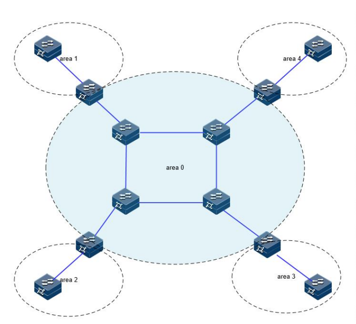
图 5-33 OSPFV3 区域划分
