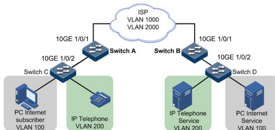
图 4-7 灵活 QinQ 应用组网示意图
