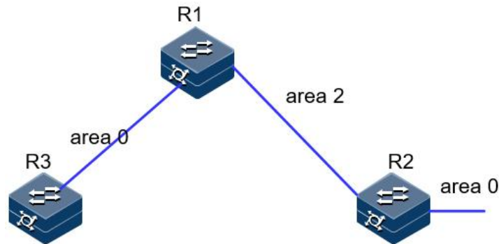
图 5-44 配置 OSPFV3 虚连接的组网图
