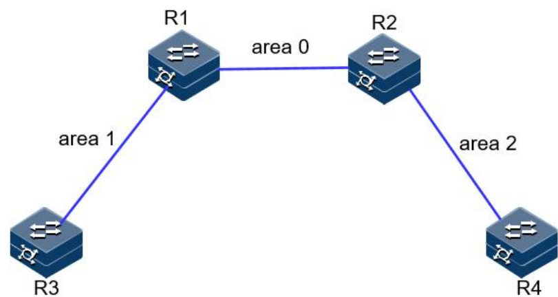
图 5-40 OSPFV3 STUB 区域示例组网图
