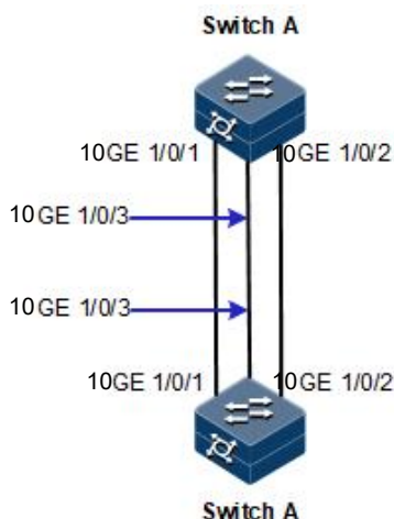
图 11-1 静态 LACP 方式链路聚合应用组网示意图
