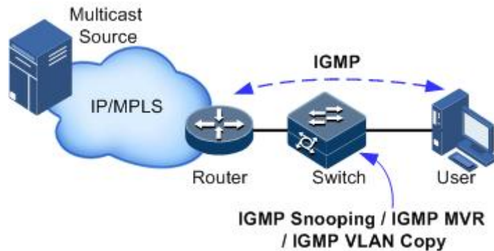
图 8-4 IGMP 和二层组播特性运行位置示意图
