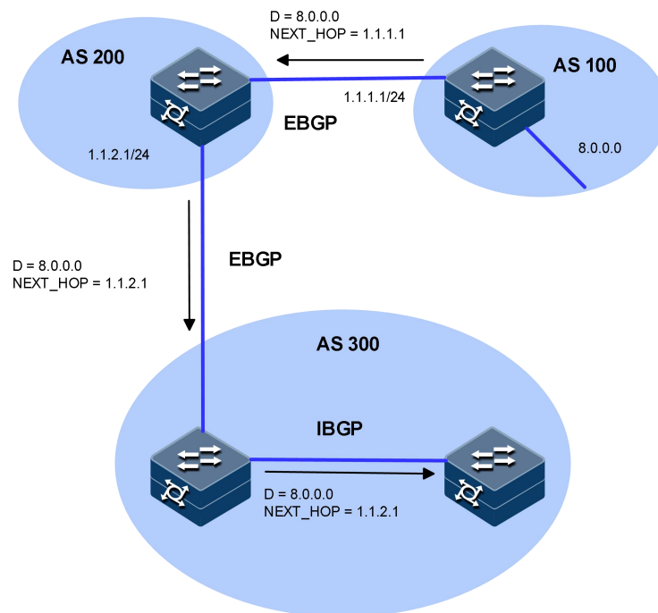
图 5-7 NEXT_HOP 属性
