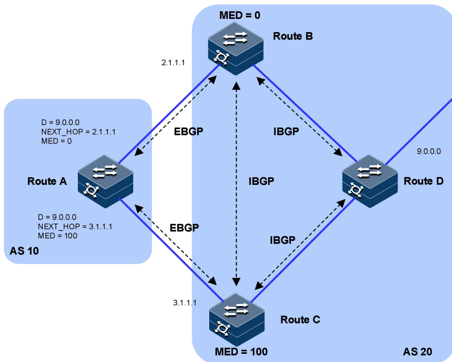
图 5-8 MED 属性
