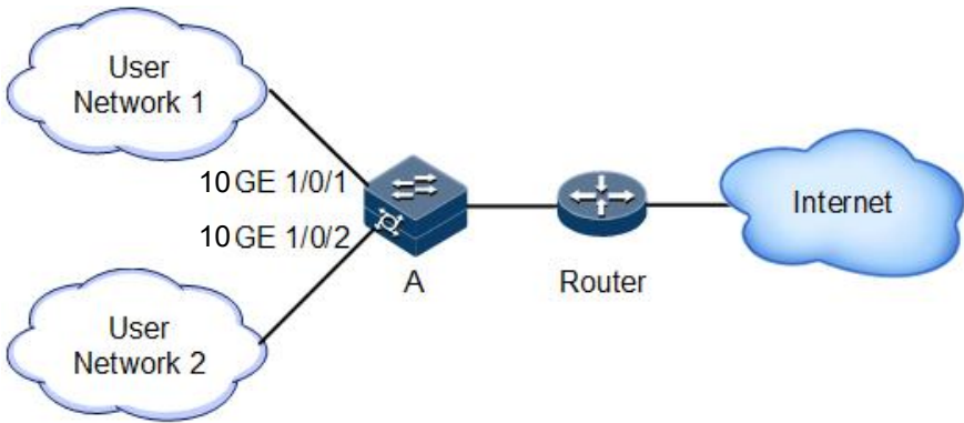
图 10-1 ACL 示例
