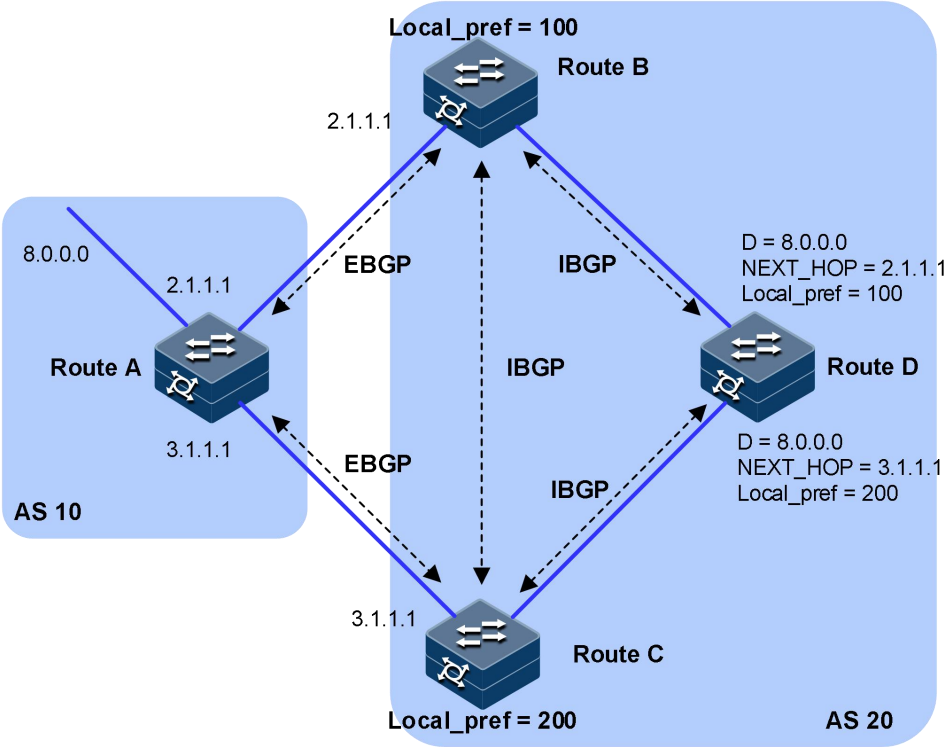
图 5-9 LOCAL_PREF 属性
