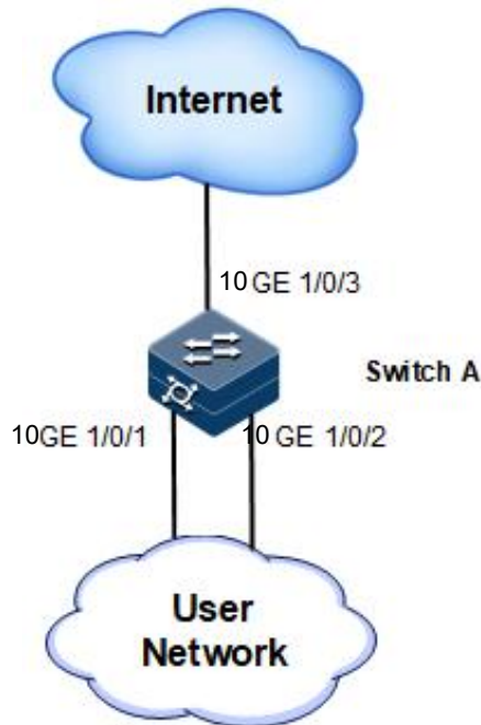
图 11-17 环路检测内环应用组网示意图
