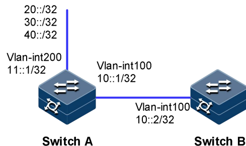
图 5-50 ipv6 路由引入中应用路由策略组网图
