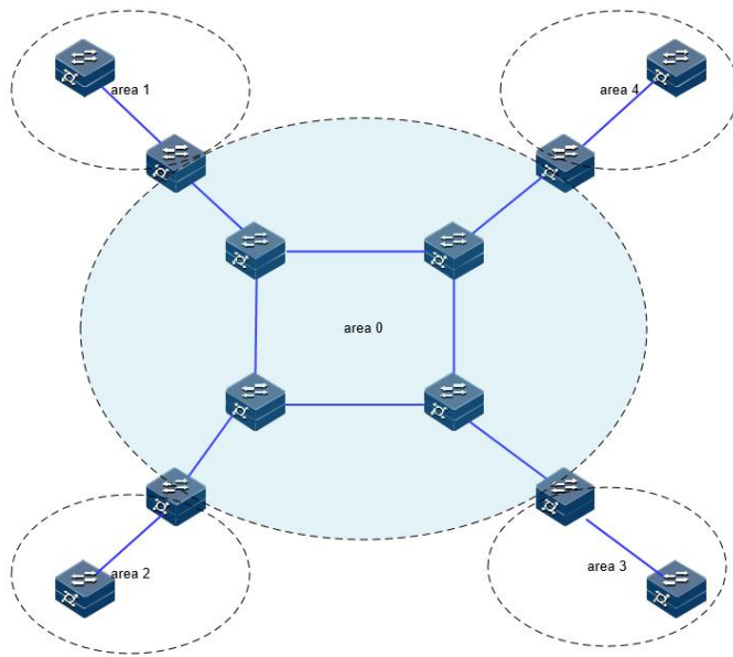
图 5-20 OSPF 区域划分
