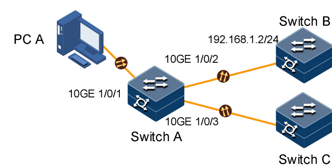
图 5-5 配置策略路由组网示意图
