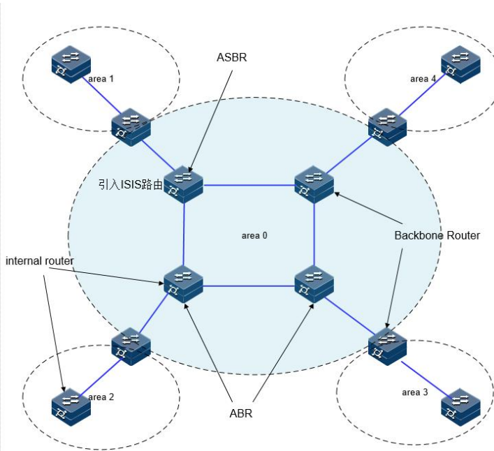
图 5-34 OSPFV3 路由器类型示例
