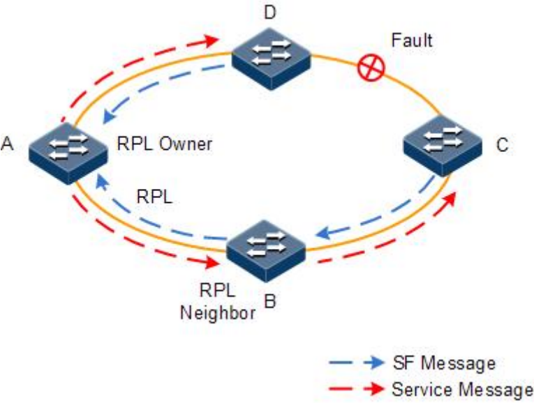
图 11-4 环网保护状态
