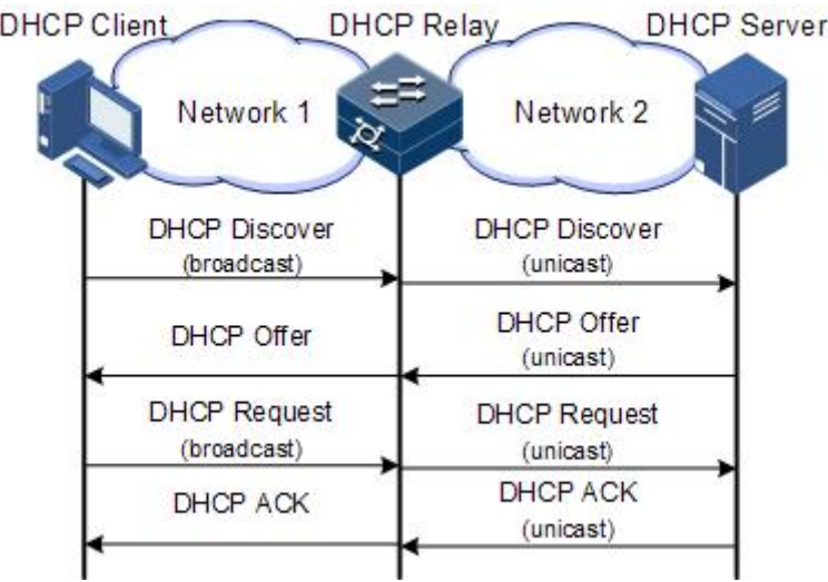
图 6-8 DHCP Relay 工作原理示意图
