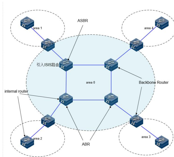
图 5-21 OSPF 路由器类型示例
